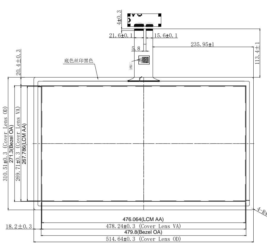
正视图
