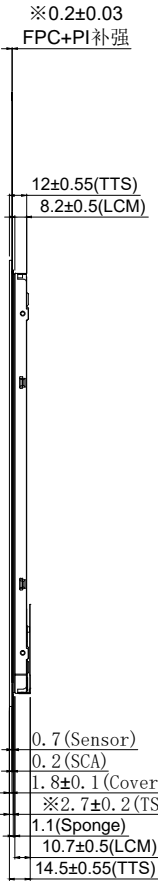
侧视图
